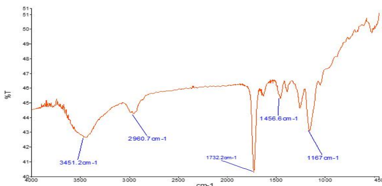
شکل (۶): طیف مادون قرمز پلیمر دیلتیازم
