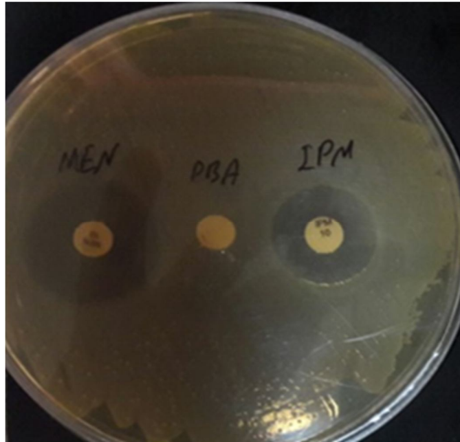
شکل (۲): تعیین فعالیت متالوبتالاکتامازی و کارباپنمازی به روش سینرژیزم دیسک دوتایی
