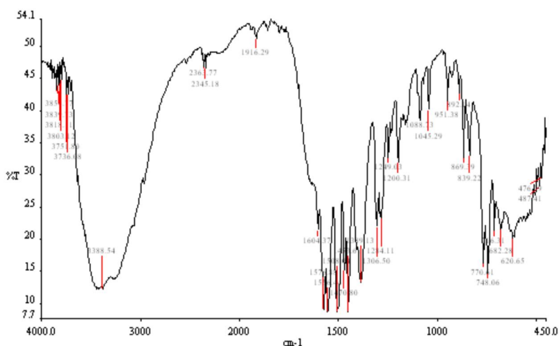
تصویر (۲): طیف FTIR، PAMAM قبل از الکتروسی
