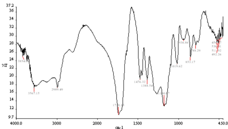
تصویر (۳): طیف FT-IR، داکسوربیسین قبل از الکتروسی
