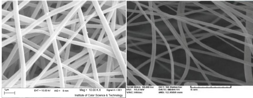
شکل (۱): یک نمونه تصویر SEM از نانو فیبرهای تولیدشده طبق الگوی جدول (۱)، ردیف سوم (۱۹)
