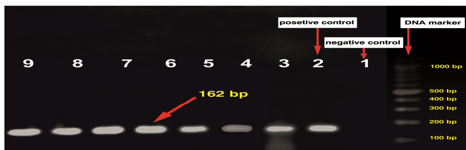
شکل شماره (۲): الکتروفورز ژل آگاروز ۱ درصد برای محصول تکثیر یافته ژن mecA (قطعه ۱۶۲ جفت بازی) به وسیله PCR ردیف ۱: کنترل منفی ردیف ۲: کنترل مثبت ATCC ۷۰۶۹۸ ردیف ۳ تا ۹: سویه‌های بالینی
